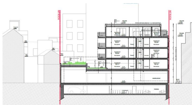
Doorsnede dwars op de Zeehondstraat - ontwerp. Uittreksel uit het aanvraagdossier
