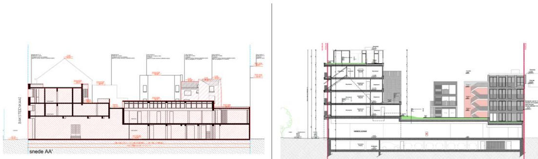
Langsdoorsnede ter hoogte van nr. 38-40 : bestaande en ontworpen toestand –documenten uit het aanvraagdossier
