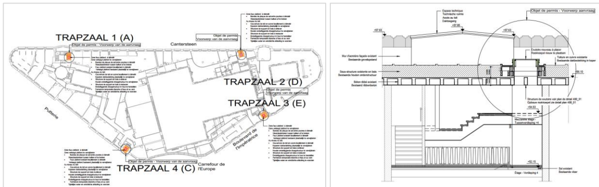
Inplanting van de rookkoepels en type doorsnede van de rookkoepels boven de betreffende trapzalen (documenten uit het aanvraagdossier)
