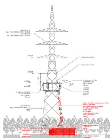
Vue en coupe de l'installation. Extrait du dossier.
