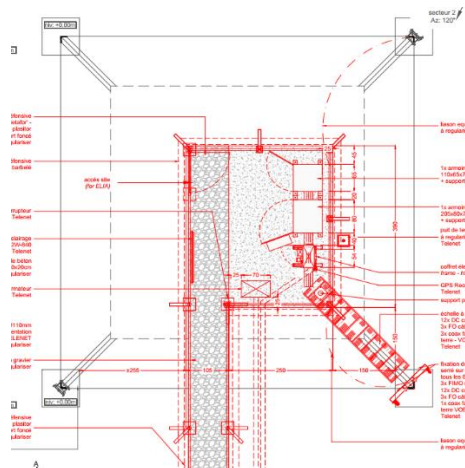
Implantation de l'installation. Extrait du dossier.
